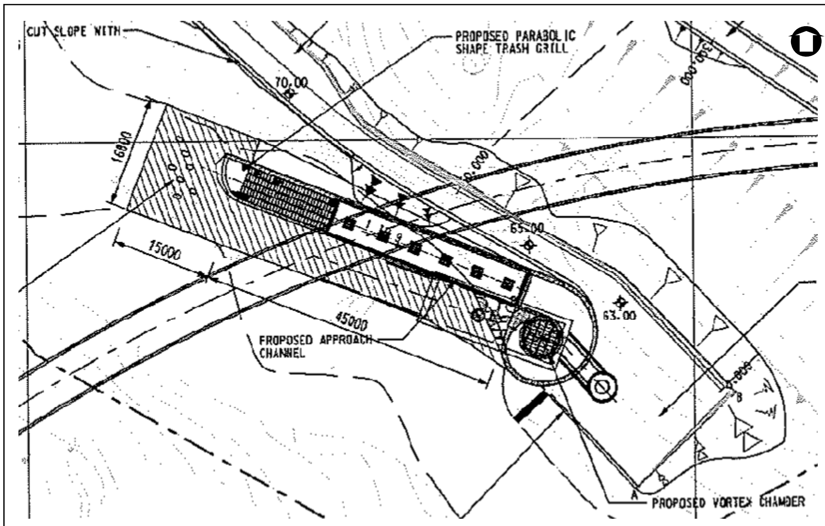
Figure 3 : Works of Intake I-3 at Tso Kung Tam Stream 圖 3: 位於曹公潭的收水口I-3工程圖
